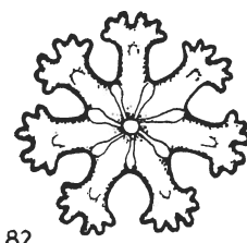
FIG. 82 — Discoaster bronnimanni nov. spec. Ans d. Facies inferior. x 1800 etwa.
