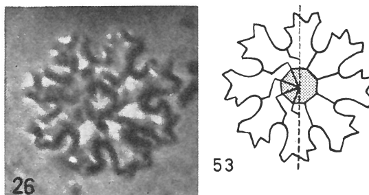
Figs. 26, 53 — Discoaster monstratus n. sp., Holotypus, SM. B 9582 (D 40.5/124.0). Donzacq, Carrière de la Tuilerie; Lutetien inférieur. 53) Schema eines 8-strahligen Stückes. Linke Hälfte: Verlauf der verbindungsnahte auf der Oberseite. Rechte Hälfte: Verlauf der Verbindungsnahte auf der Unterseite. Lutetien inférieur. Vergr. einheitlich x 2000.
