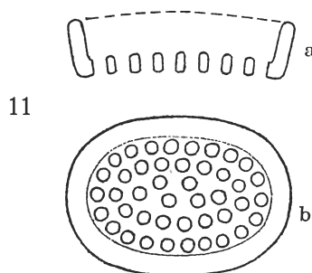
Fig. 11 — Discolithus raclus nov. spec. a) vertikaler Längsschnitt, b) Oberseite. x 3000.
