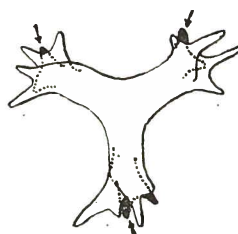
FIG. 2 — Marthasterites furcatus (DEFL.) var. bramlettei n. v. Holotype. BZ 24. Santonien, marne de Bonham, Detroit, Texas, U.S.A. x 3200.
