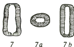
FIGS. 7, 7a, 7b — Nannoconus planus n. sp., 7) longitudinal section (large axis); 7a) cross section; 7b) longitudinal section (small axis); x 2000.
