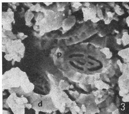
Fig. 3 — Sollasites pristinus n. sp., holotype, restes d'une coccosphère: coccolithes sur leurs faces proximale (p), distale (d). Toarcien, Ancerville. x 10.000 env. (n° 6627).
