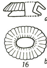
FIG. 16a, b — Tremalithus amplus , x 3000. a) in aufrechter Stellung. Die linke Hälfte bietet die Seitenansicht, die rechte Hälfte den aufrechten Längsschnitt des Objektes. b) An- sicht der Oberseite.
