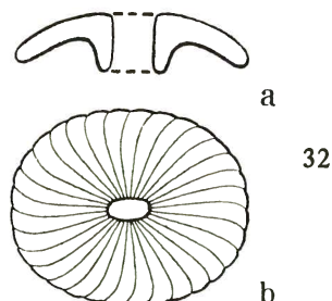
FIG. 32a, b — Tremalithus honestus nov. spec. a vertikaler Längsschnitt, b Oberseite. x 3000.
