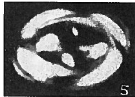
Fig. 5 — Arkhangelskiella inclinata n. sp. Holotypus. x 3000.
