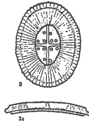
FIGS. 3, 3a — Arkhangelskiella parca n. sp., 3) plan view, 3a) side view; x 4000.
