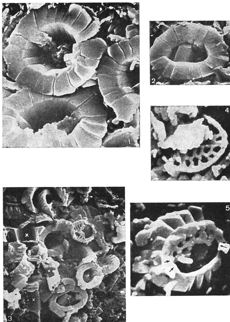
Figs. 1-5 — Calyculus cribrum n. gen. Toarcien inférieur, « schistes carton » de Lorraine. 1) Holotype, restes d'une coccosphère (coccolithes vus par leur face distale). Fécocourt. x 6.500 env. (n° 6049). 2) Face distale; un gros cristal de calcite barre l'aire centrale. Ancerville. x 6.500 env. (n° 6657). 3) Divers exemplaires cassés transversalement (x); on remarquera la profondeur de la zone centrale. Fécocourt. x 3.300 env. (n° 5760). 4) Grille détachée du reste du coccolithe. Ancerville. x 13.500 env. (n° 6659). 5) Face proximale; on remarquera la forme des éléments (→) constituant la ceinture basale. Ancerville. x 13.500 env. (n° 6654).
