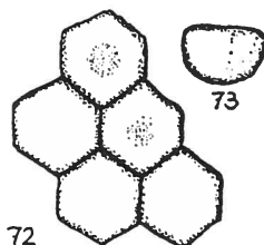
FIGS. 72, 73 — Favolithora cyclopia nov. gen., nov. spec. — 72: Ansicht eines Wandstückes. 73: Seitenansicht eines Einzelsteines. x 1800 etwa.
