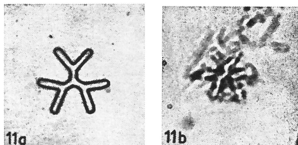
Figs. 11a, b — Discoaster bramlettei n. sp. x 2000 einh. a) Schema. b) Holotypus, SM.B 8170. — Repke 1: 371.8–380.3 m K. 2; unteres Ober-Eozän.
