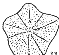
Fig. 33 — Discoaster slatiorensis n. sp.
