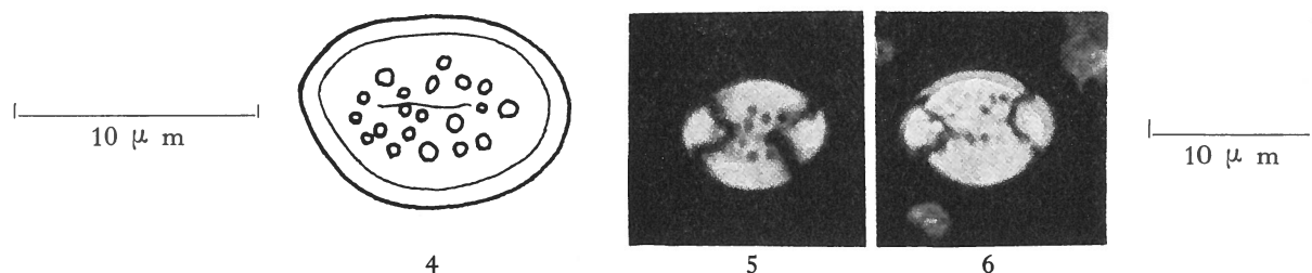
Figs. 4-6 — Discolithina enormis sp. n., 4, 5) Holotyp, Bhg. Nennhausen, Oberoligozän; 6) Paratyp, Bhg. Setzin 4/63, Pröp. 175 (50.0/18), Obermiozän.
