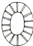
Fig. 7 — Discolithus constans n. sp. x 1350.
