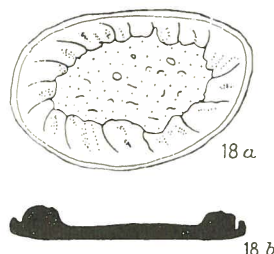
FIGS. 18 a, b — Discolithus coronatus n. cent., a) vue apicale, b) coupe axiale. x 5000 env.
