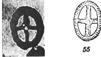
Figs. 4, 55 — Discolithus crux n. sp., 4) \times 5,600 . Marne lutétienne, Donzacq, Landes.
