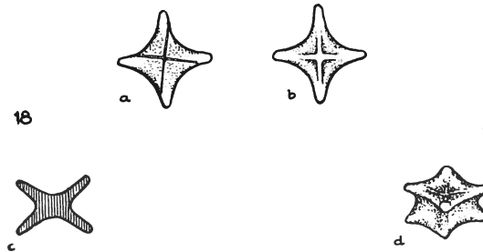
Fig. 18a-d — Nannotraster concavus n. sp. a) Facies superior; b) Facies inferior; c) Querschnitt; d) Seitenansicht, schräg. \times 1900 .
