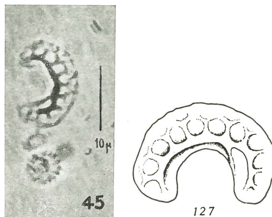
FIG. 45 — Peritrachelina ornata n. g. n. sp. Eocène, Lutétien. x 1560. FIG. 127 — Peritrachelina ornata DEFL. (Lutét., Donzacq) AV 11. x 3600. (1954).
