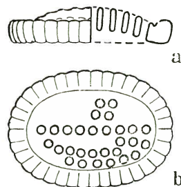
FIG. 26 — Pontosphaera cribrosa nov. spec. a linke Hälfte: Ansicht der Breitseite — rechte Hälfte: vertikaler Längsschnitt, b Oberseite. x 3000.
