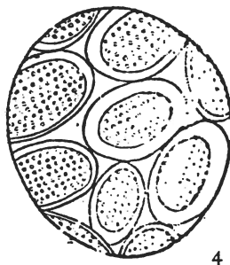
Fig. 4 — Ponthosphaera discopora SCHILLER, x 1800. Boden der Discolithen mit zahlreichen Poren versehen.
