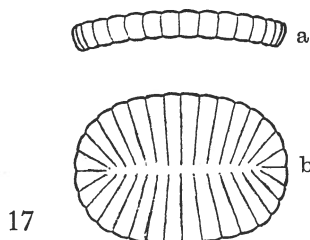
Fig. 17 — Pontosphaera gareta nov. spec., a) Breitseite, b) Oberseite. x 3000.
