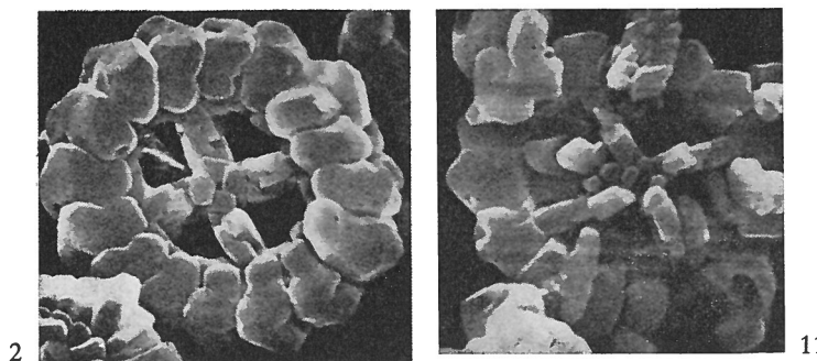
Figs. 2, 11 — Prediscosphaera serrata n. sp. 2) Allotype: Face proximale. Campanien supérieur d'Arpenty (profondeur 83 mètres). Cliché S. 1828. x 7 650 environ. \alpha = 45^\circ . 11) Holotype: face distale. Campanien inférieur d'Arpenty (profondeur 83 mètres). Cliché S. 1857. x 5 700 environ. \alpha = 0^\circ .
