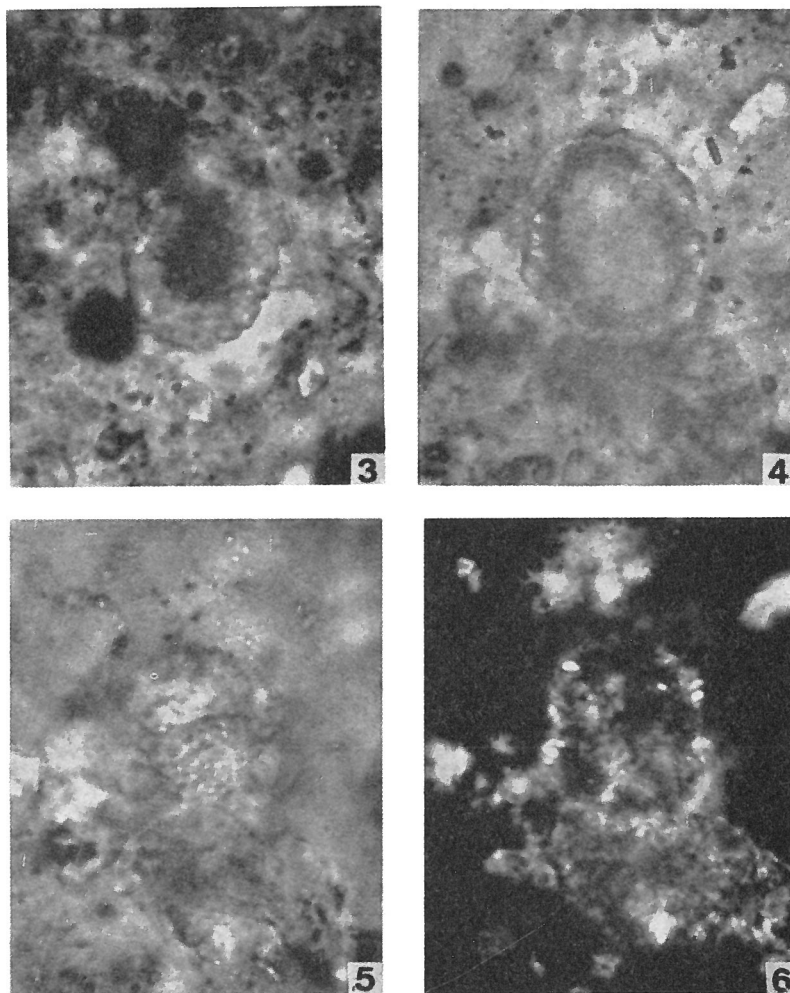
Figs. 3-6 — Coccolithites fallax n. sp.; 3) paratype, 4-6) holotype, (5) surface centrale, (6) lumière polarisée. x 1540.
