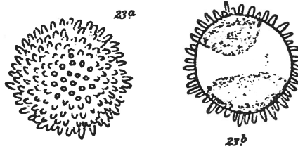
Fig. 23 a, b - Rhabdosphaera brevispina n. sp.
