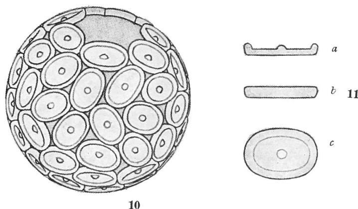
Figs. 10, 11 — Syracosphaera catillifera nov. spec. 10) Schale, x 3750. 11 a-c) Coccolith, x 6000, (a) Längsschnitt, (b) Seitenansicht, (c) Draufsicht.
