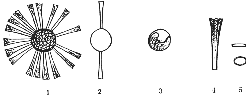
Figs. 1-5 — Thorosphaera elegans n. sp. 1) Ganze Zelle, von oben (von der Fläche) gesehen, 2) Schematischer Durchschnitt einer Zelle, 3) Der Zelleib mit Chromatophoren, lichtbrechenden Körpern und Kern, 4) Ein röhrenförmiger Coccolith, 5) Ein scheibenförmiger, von der Fläche und von der Seite gesehen.
