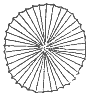
Fig. 13 — Tremalithus dilucidus n. sp. x 1350.
