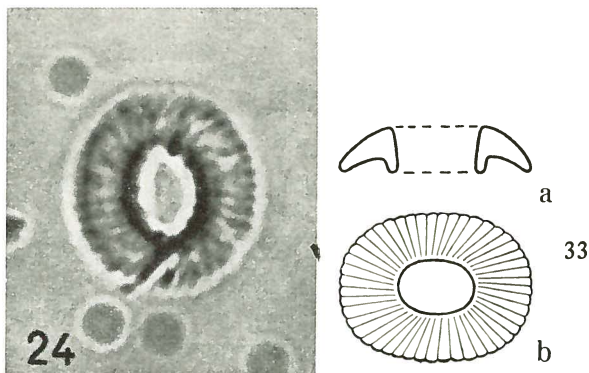
FIG. 24 — Tremalithus marginatus nov. spec. Mikrophotogramm. Oberseite. Probe 22 (Miocän). x 3000. FIG. 33a, b — Tremalithus marginatus nov. spec. a vertikaler Längsschnitt, b Oberseite. x 3000.
