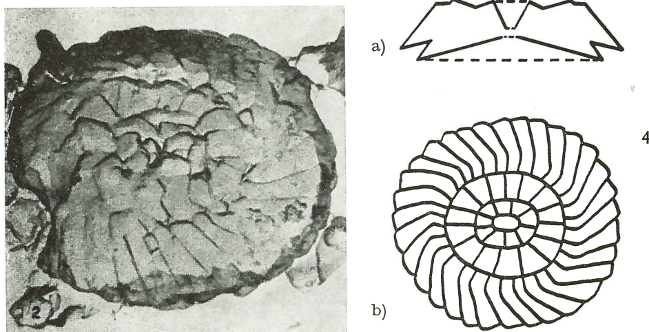
FIG. 2 — Watznaueria angustoralis n. sp. — Oberseite — 12000 x. FIG. 4a, b — Watznaueria angustoralis — a) vertikaler Schnitt, b) Oberseite — 6000 x.
